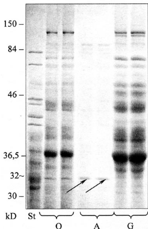
Рис. 2. Электрофоретические спектры полипептидов средней пробы семян в популяции 1 Hedysarum theinum до и после диализа. SDS-система, +Me-вариант, St — стандартный образец линии E. sibiricus (ALT-1); O — суммарный экстракт солерастворимых белков; A — альбумины; G — глобулины
