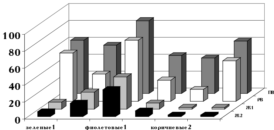
Рис. 3. Всхожесть семян и жизнеспособность проростков Hedysarum theinum в зависимости от цвета семян в двух популяциях. 1 — в субальпийском редколесье на высоте 1700 м над ур. м.; 2 — на альпийском лугу на высоте 2100 м над ур. м. ПВ — всхожесть за 3 дня (энергия прорастания); РВ — всхожесть за 10 дней; Ж1 — жизнеспособность проростков через неделю после посадки в грунт; Ж2 — жизнеспособность проростков через 2 недели после посадки в грунт
