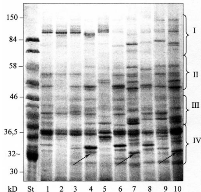
Рис. 1. Электрофоретические спектры полипептидов отдельных семян, различающихся по цвету кожуры, в популяции 1 Hedysarum theinum .
