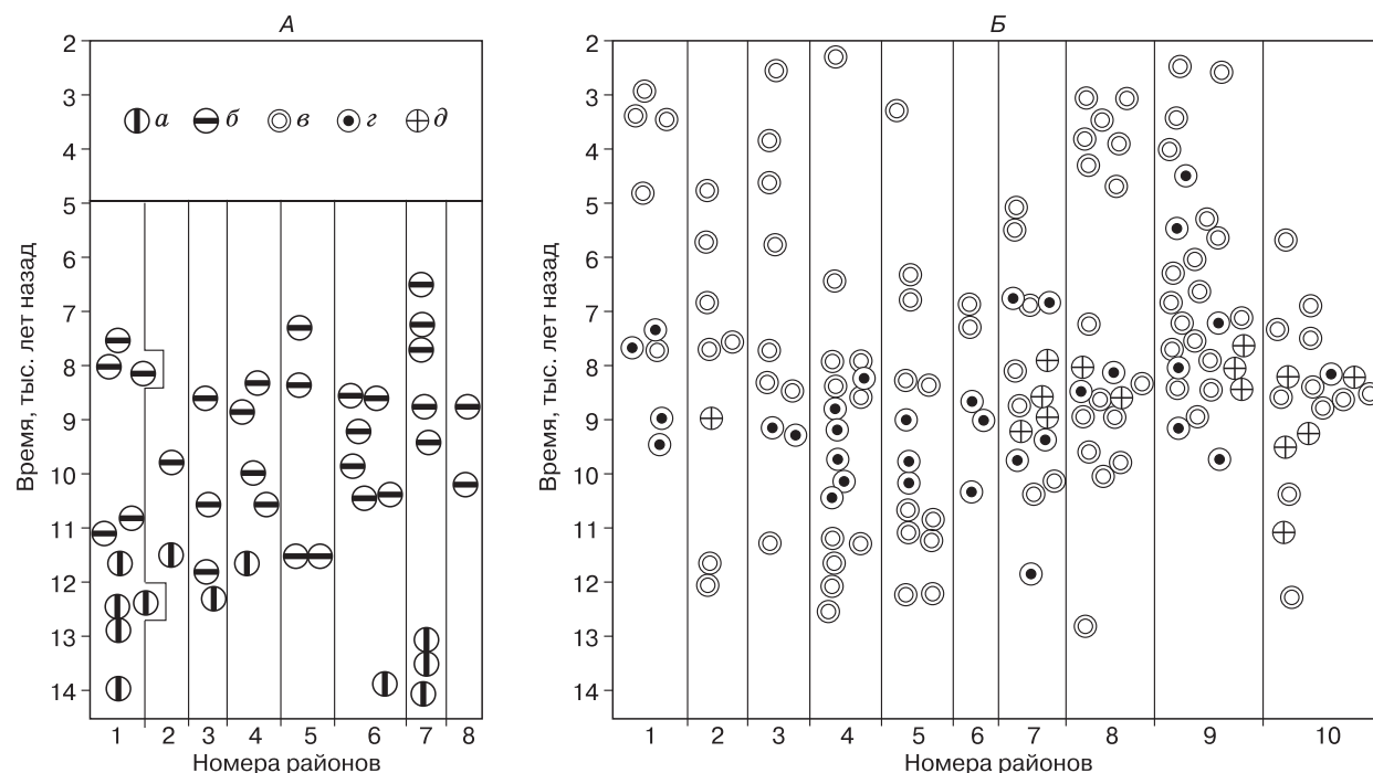
Рис. 5. Радиоуглеродные даты (некалиброванные) на едомах (А) и в аласах (Б).
