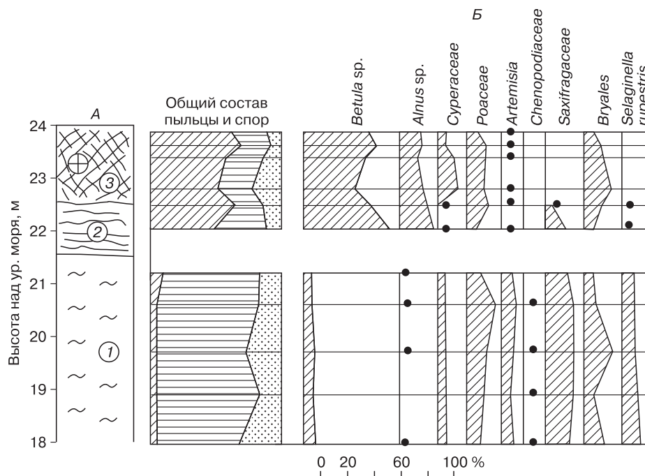
Рис. 7. Спорово-пыльцевая диаграмма верхней части разреза аласа в обнажении Станчиковский яр на р. Малый Аной (фрагмент, аналитик Н.О. Рыбакова).
