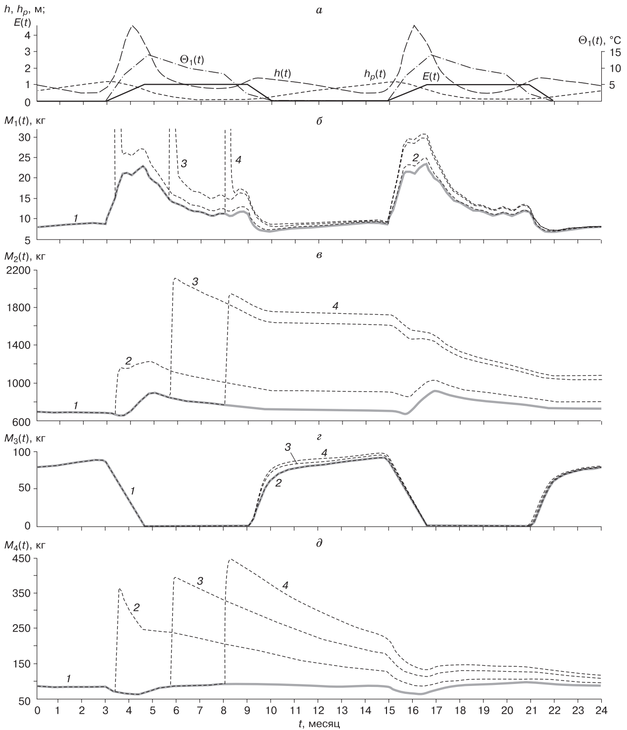
Рис. 3. Основные гидрометеорологические характеристики модели и динамика загрязненности кумулятивных зон.
