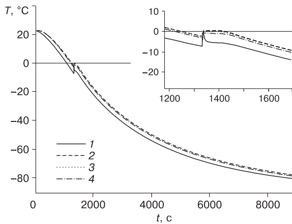
Рис. 4. Зависимость температуры ( T ) от времени ( t ) охлаждения для термодпар (Т1–Т4), установленных на разных глубинах в образце из увлажненного песка:
