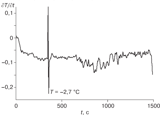
Рис. 5. Зависимость первой производной по температуре ( \partial T/\partial t ) для одной из термодпар от времени ( t ) для образца из древесины.
