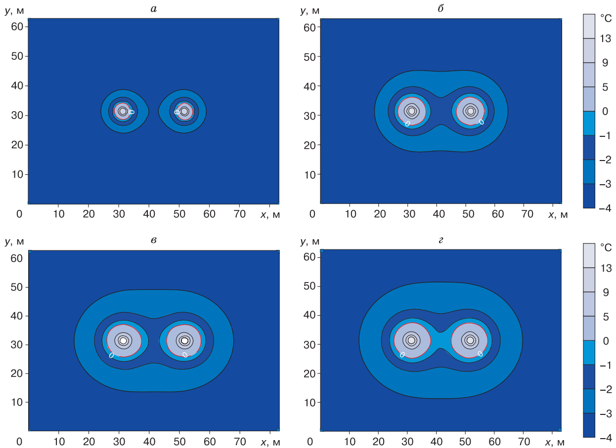
Рис. 3. Температурное поле в горизонтальной плоскости на глубине 5 м для различных моментов времени: а – 1 год, б – 10 лет, в – 25 лет, г – 50 лет.
