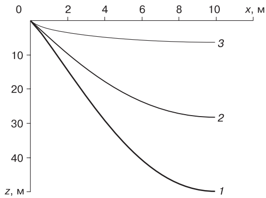
Рис. 2. Граница протаивания в плоскости двух скважин, полученная с помощью метода последовательной смены стационарных состояний (левая половина промежутка между скважинами): 1 – 25 лет, 2 – 30 лет, 3 – 40 лет.
