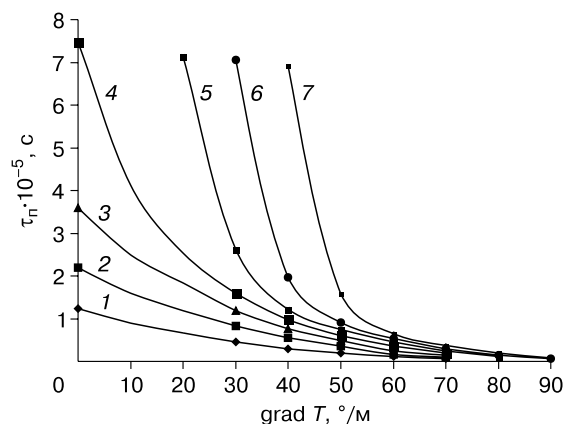
Рис. 1. Семейство зависимостей продолжительности предкристаллизационного переохлаждения влагоненасыщенной супеси \tau_n от градиента температуры \text{grad } T в приповерхностной зоне охлаждения и температуры переохлаждения T_n на внешней поверхности образца:
